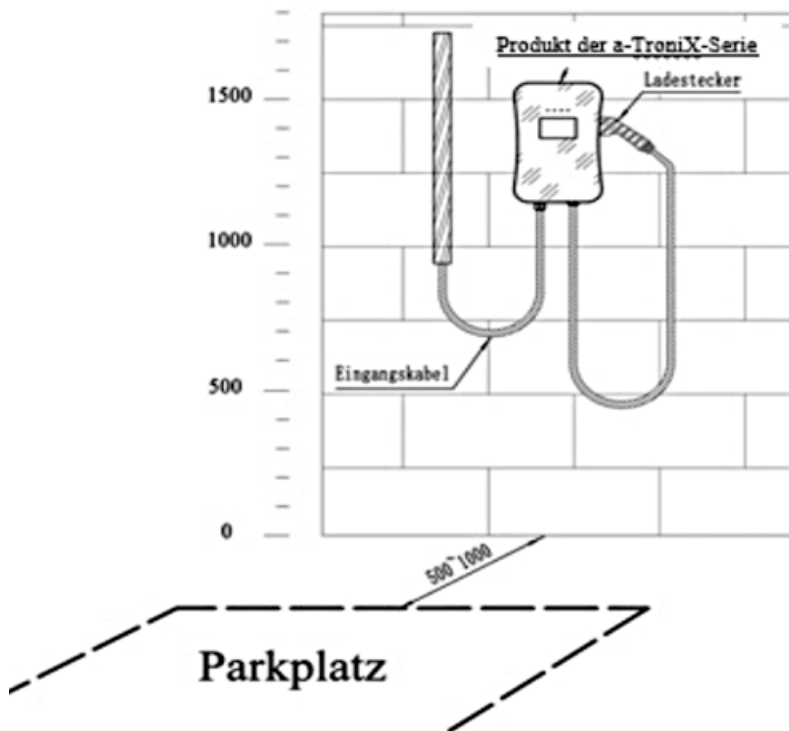
Abb. 5-1 Montieren Sie das Produkt der a-TroniX-Serie an der Wand
