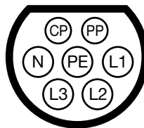
(b) 3-phasen Type 2 Buchse
