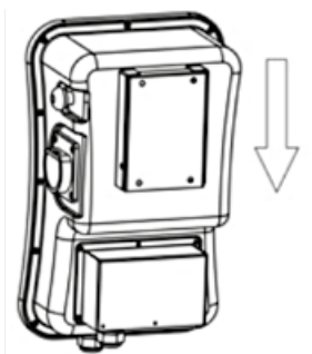
Abb. 5-4 Hängen Sie die Wallbox an den Aufsatz
