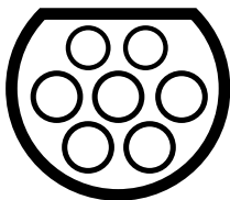
(a) Type 2 Stecker
